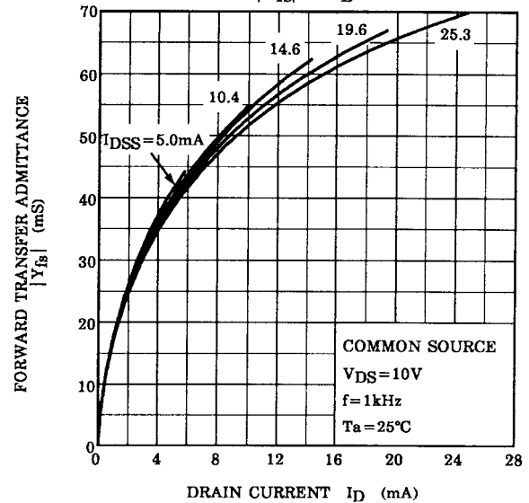
|Y_{fs}| - I_D
